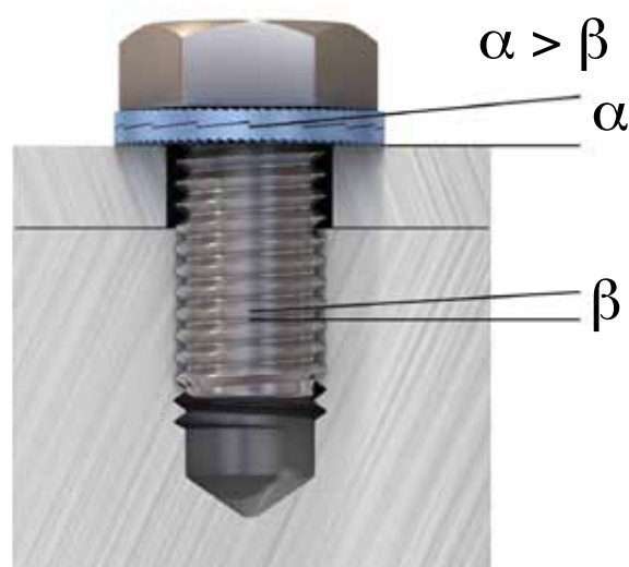
ノルトロックのウェッジロック機構
