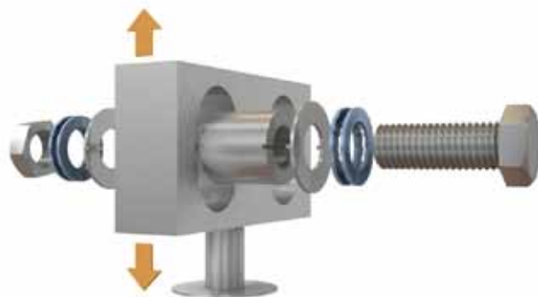
図2: 試験装置 組立部が垂直方向に振動し、ボルト締結部には、振動サイクルごとに2回の衝撃が与えられます。衝撃はボルトに対し平行です。矢印は、試験中の振動方向を示しています。試験後、締結部の回転角度を検査します。
